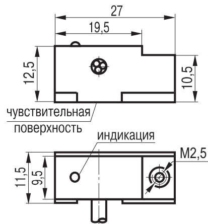
Габаритный чертёж
